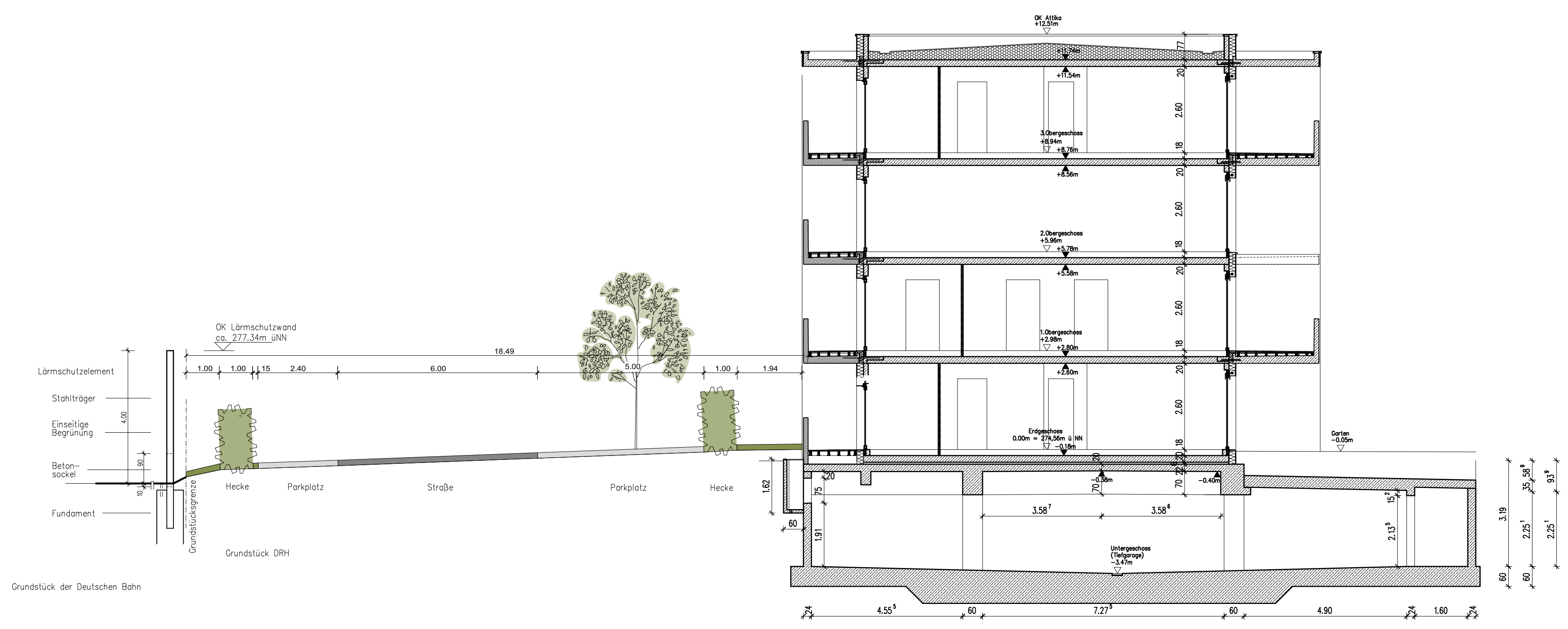
SCHNITT
